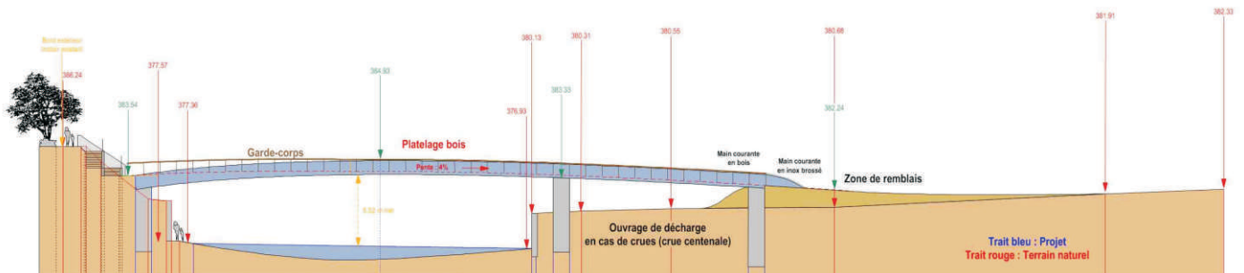
Passerelle (60 m de long) et rampe PMR en encorbellement
